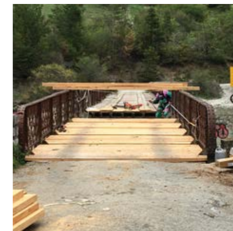
Réfection tablier Pont de Méouilles
